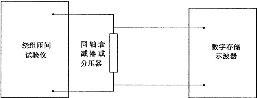
图 2 绕组匝间试验仪输出冲击电压峰值和波前时间测量线路
