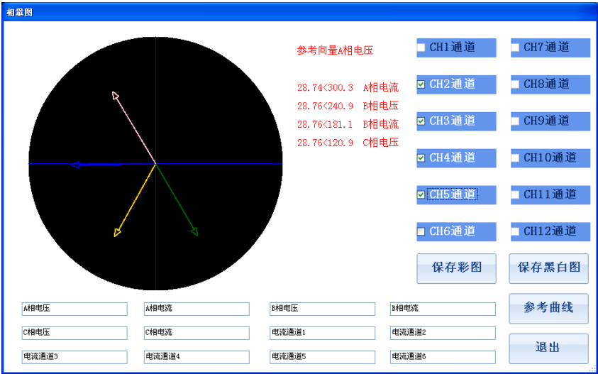
图 29 相量图工具
