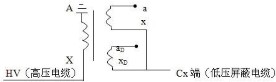
图 9 末端加压法接线
