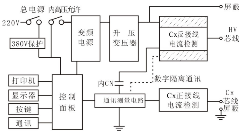
图 2 仪器结构图
