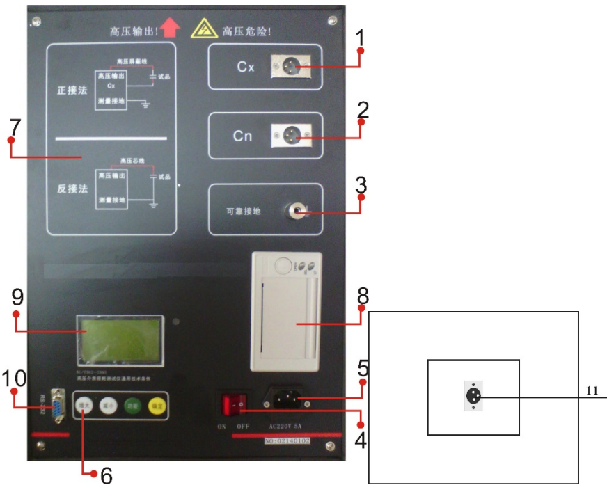
图 1 仪器面板和侧面
