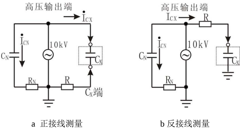
图 3 测量原理图
