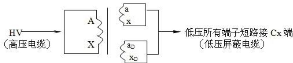
图 7 常规接线法
