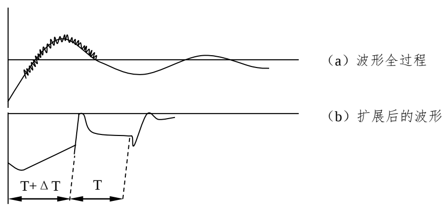
图 5 冲击高压法波形图
