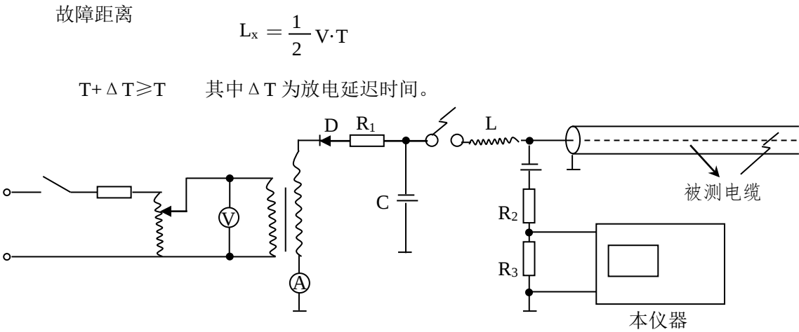
图 4 冲击高压法测试原理图
